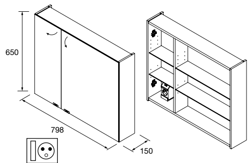
Armoire ALLIANCE 800 2 portes miroir double avec interrupteur et prise 798 x 650 x 150 mm 24062 559 €
