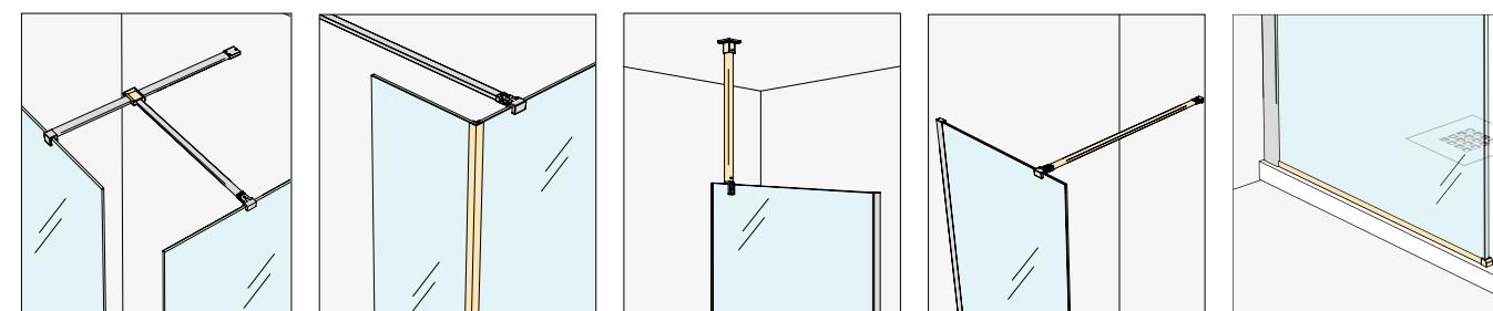
Kit de connexion entre 2 tendeurs Profilé d'angle Tendeur plafond Support mural Profilé sol 1400 mm, v. Fixe 8 mm
