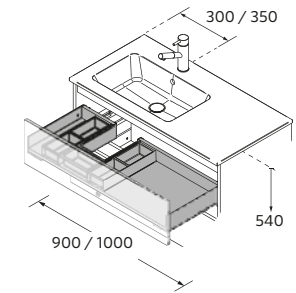
TIROIR MÉTALLIQUE HAUT POUR MEUBLE AVEC DÉCOUPE SIPHON, COQUETTE A DROITE
